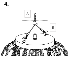
Cable eléctrico no representado para una mejor visualización. For better visualization the electrical cable has not been depicted.
