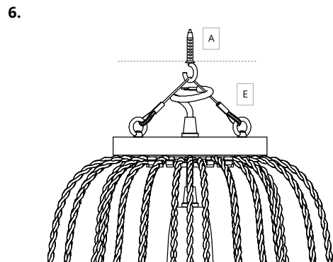
Cable eléctrico no representado para una mejor visualización. For better visualization the electrical cable has not been depicted.
