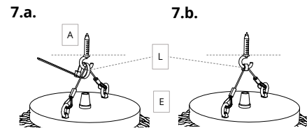
Cable eléctrico no representado para una mejor visualización. For better visualization the electrical cable has not been depicted.
